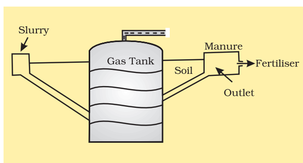
Fig. 3.21 : Biogas
